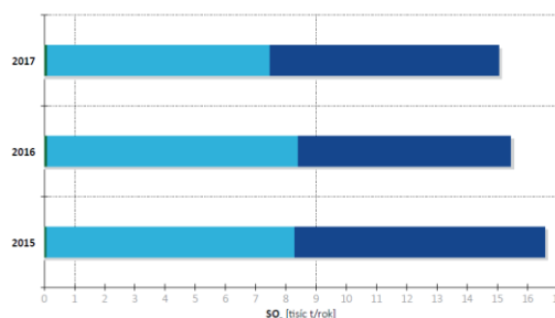
Oxid siřičitý
